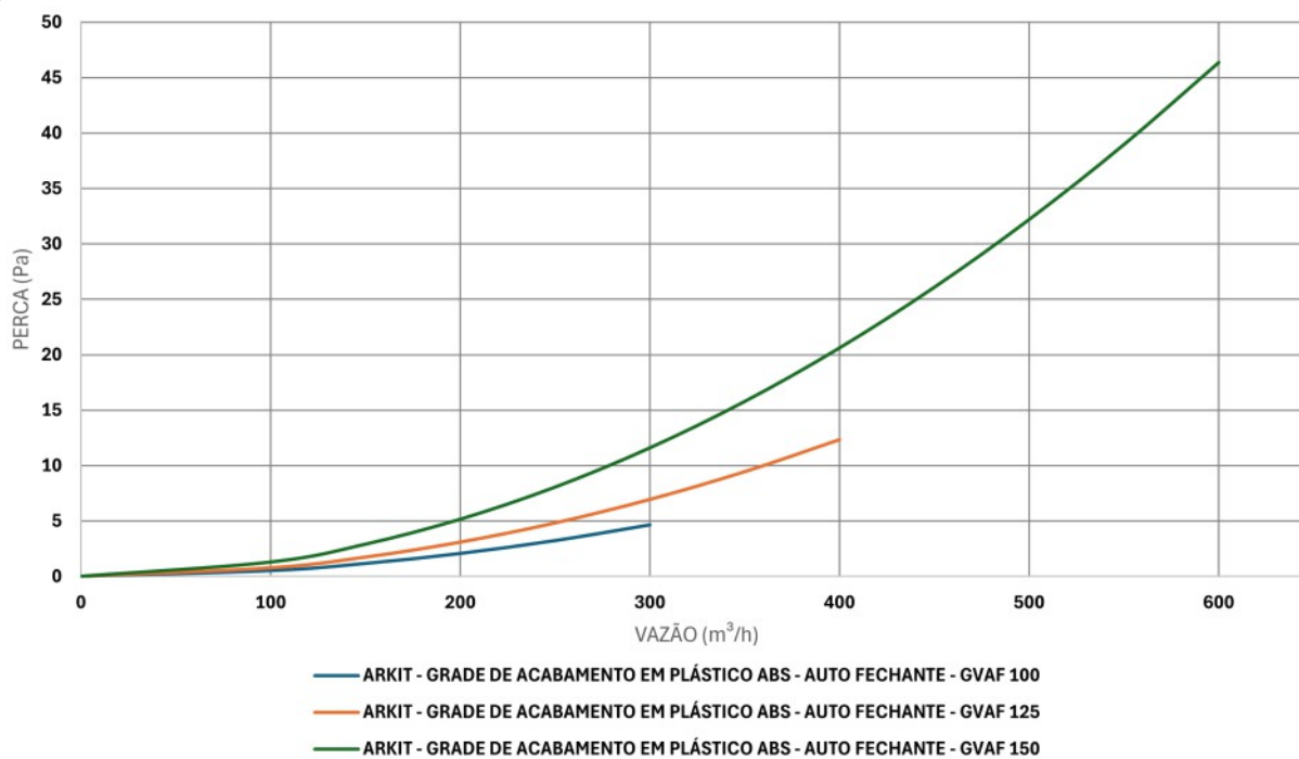
PERDA DE CARGA GRADES AUTO FECHANTES
