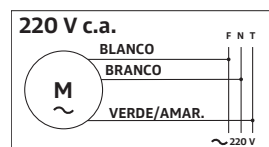
Figura 3.1: Diagrama de conexión eléctrica.
